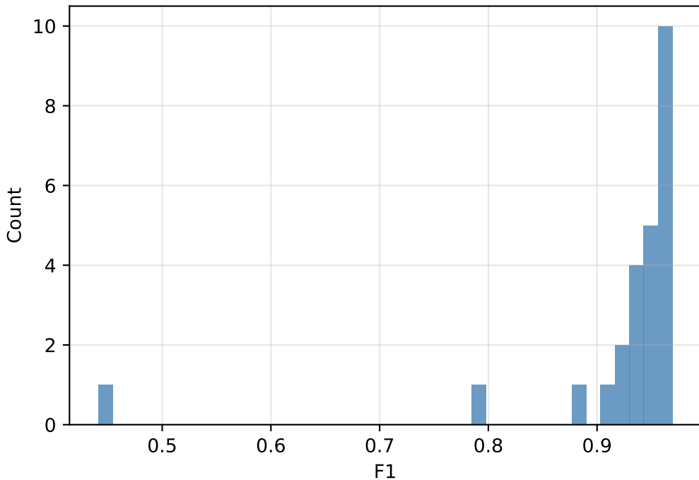
F1 Distribution
