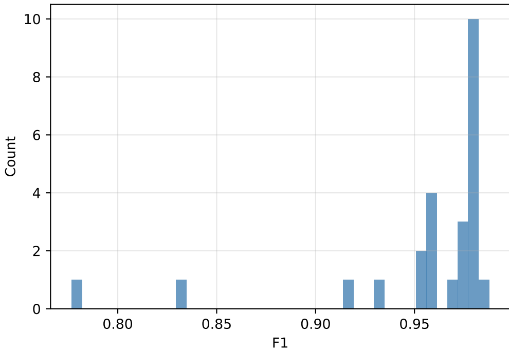
F1 Distribution
