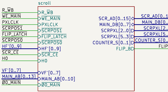
File: scroll.kicad_sch
