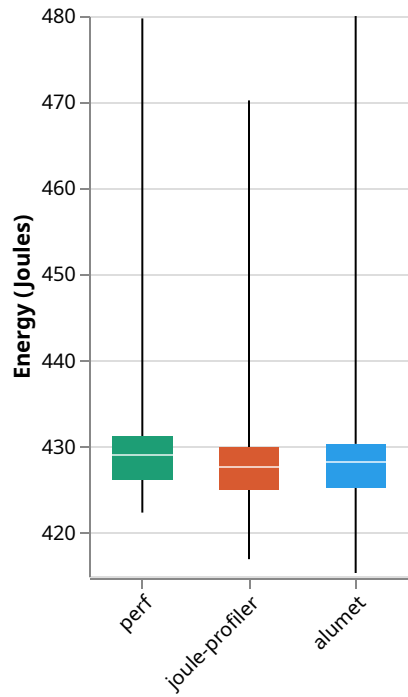
PACKAGE-0
