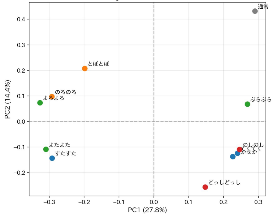
SigLIP 埋め込みのPCA
