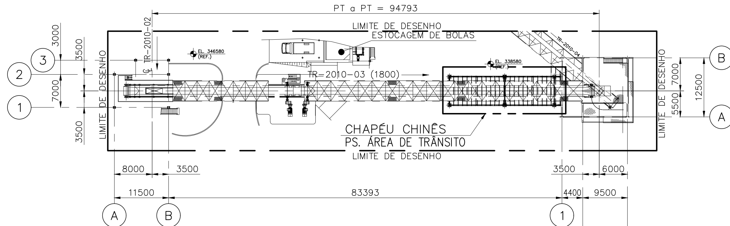
PLANTA DE LOCAÇÃO ESC. 1:500
