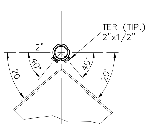
DETALHE BICOS ESC. 1:10
