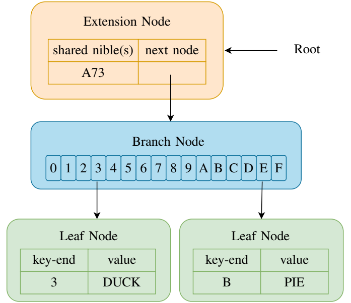
Fig. 1. Custom hexary Merkle Patricia Trie
