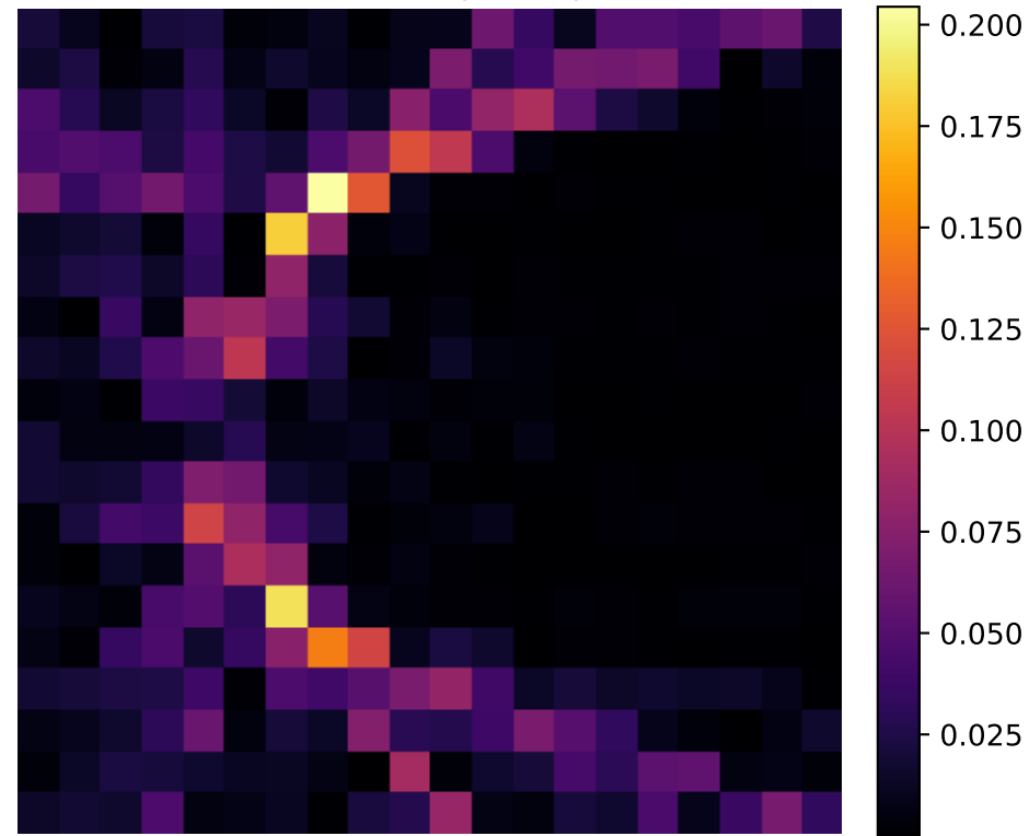
Error Map |A - B|
