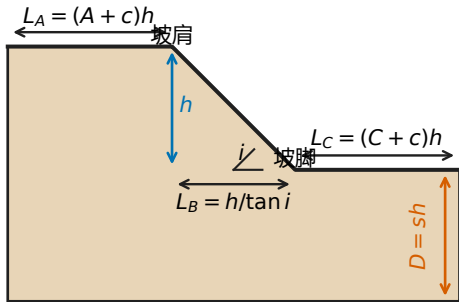
参数化坡地几何
