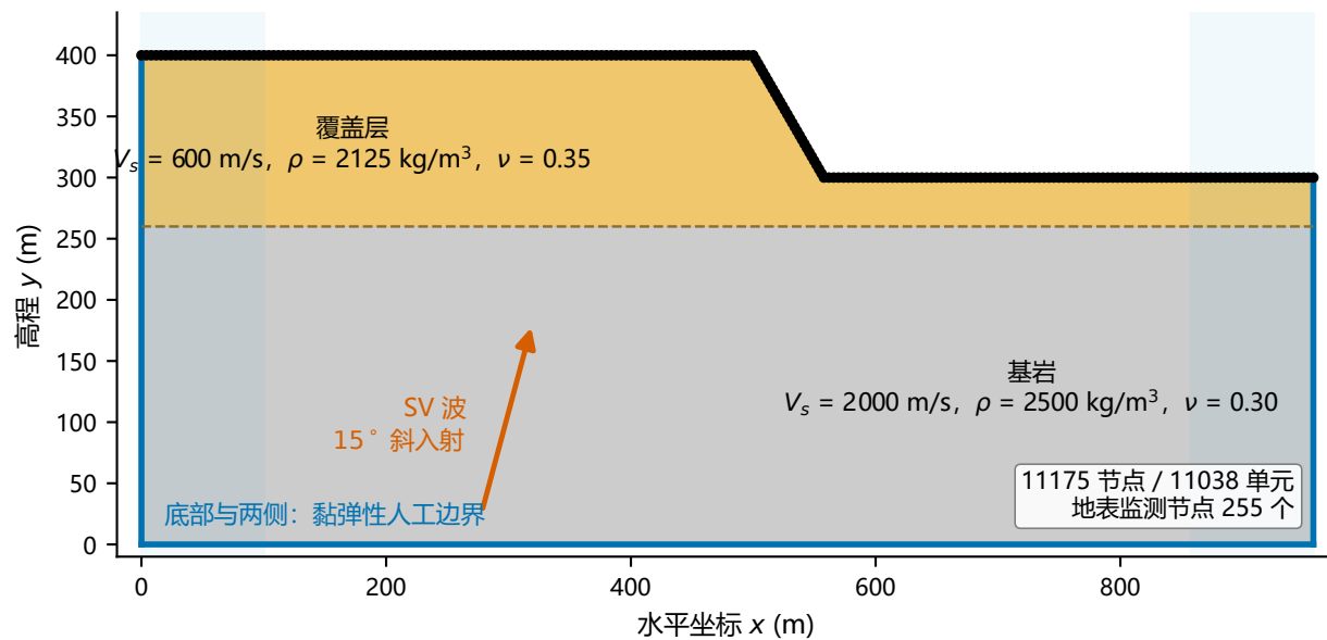
(a) P061 全域几何、材料与边界
