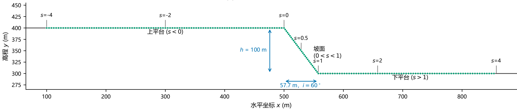
(b) 地表监测节点与归一化坐标
