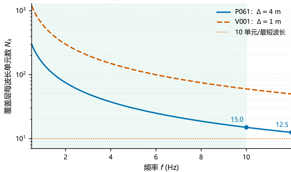
(d) 最不利覆盖层的网格分辨率
