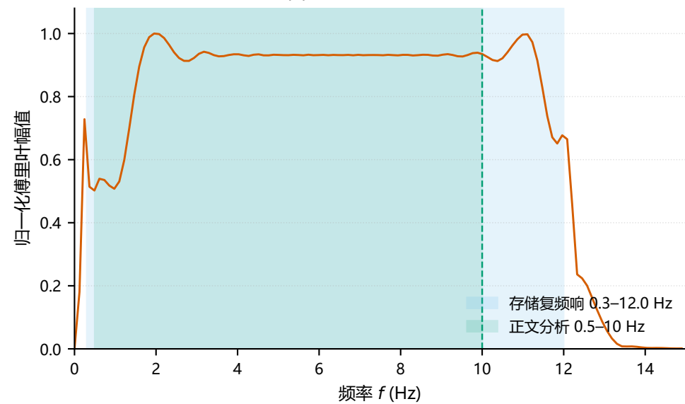
(b) 输入频谱与分析频带
