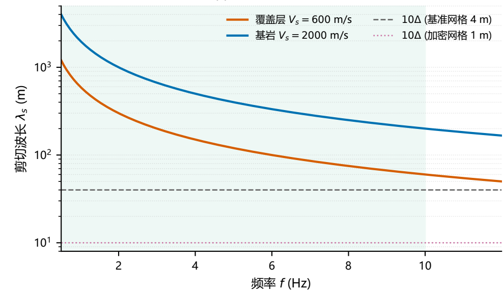
(c) 材料波长与网格尺寸
