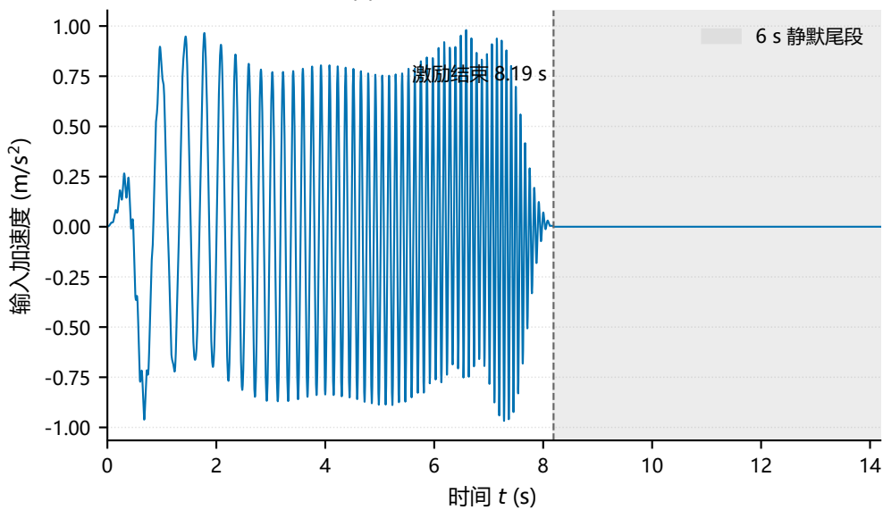
(a) G1b 宽频多正弦输入时程
