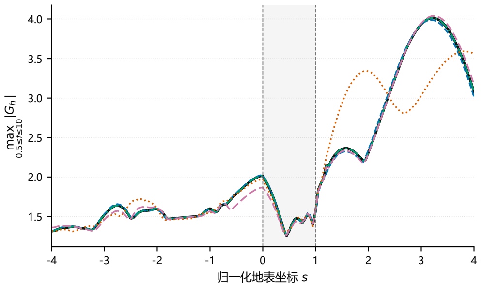
(c) 全地表频带峰值的保持性
