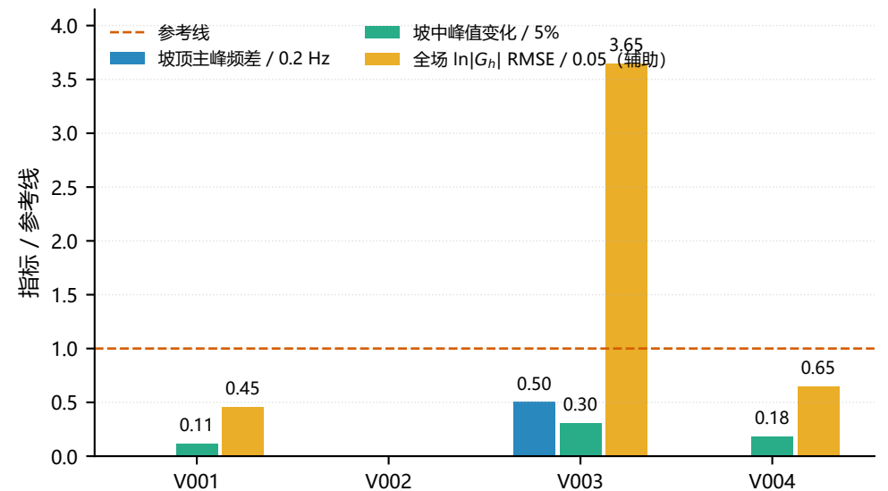
(d) 两项主要判据均满足, V003 辅助全场指标偏大
