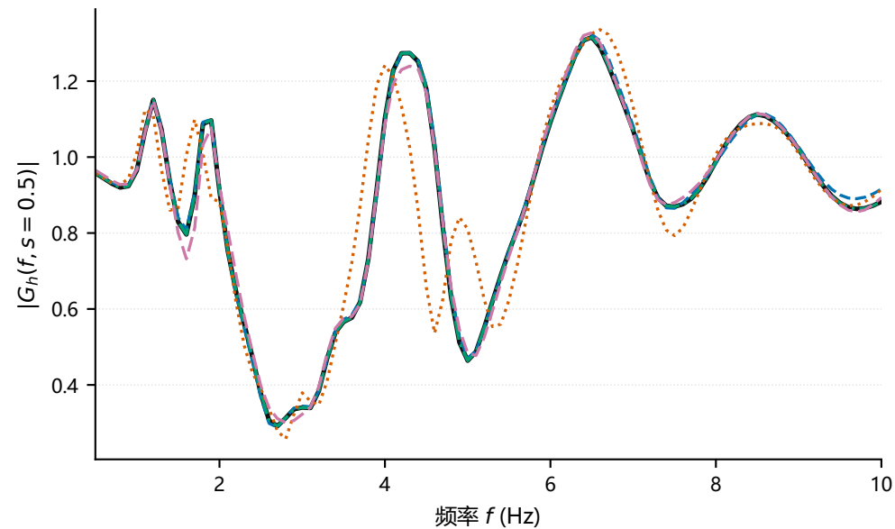
(b) 坡面中部复频响应幅值
