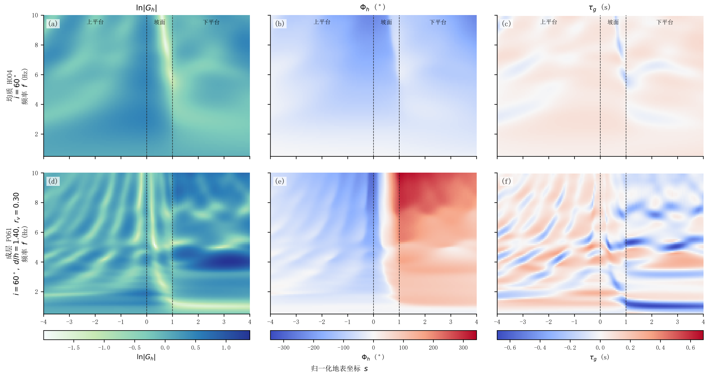
统一左侧一维自由场参考下的代表工况复频响应联合场
