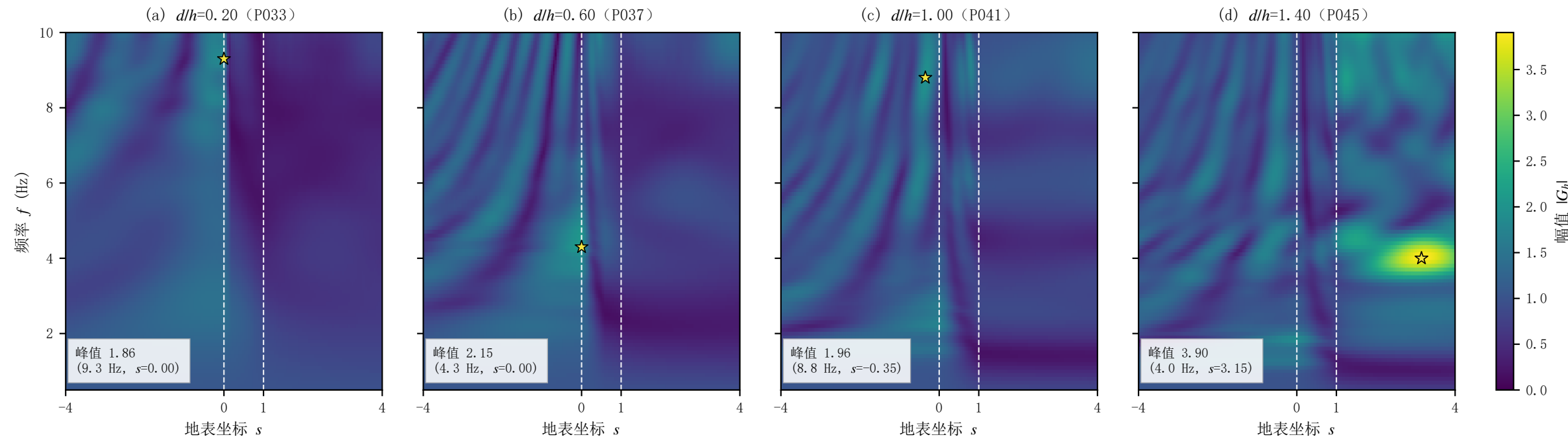
覆盖层厚度单因素对比：固定 i=45^\circ 、 r_v=0.30
