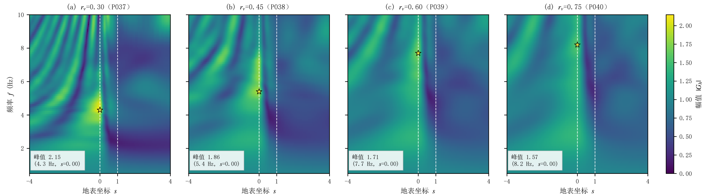
覆盖层波速比单因素对比：固定 i=45^\circ 、 d/h=0.60
