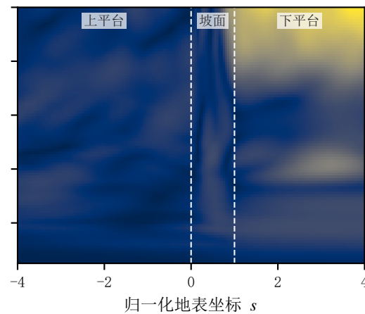
(e) 第3阶复数模态幅值
