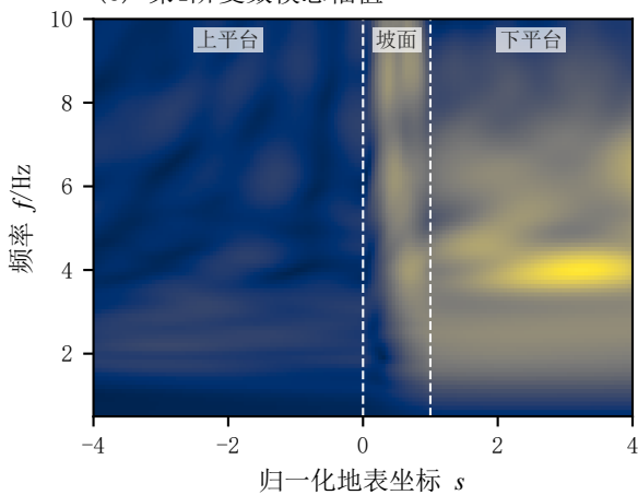
(c) 第1阶复数模态幅值
