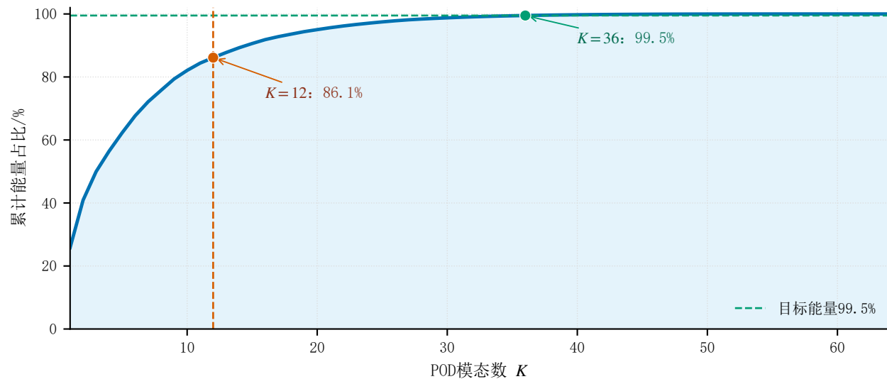
(b) 完整P组输出矩阵的POD累计能量
