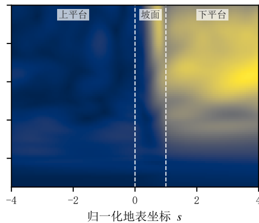
(d) 第2阶复数模态幅值
