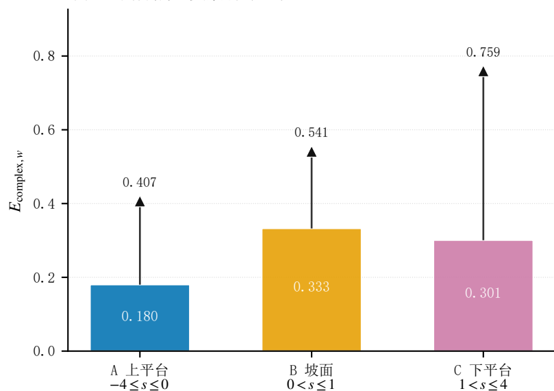
(c) 空间分层：复数场综合误差
