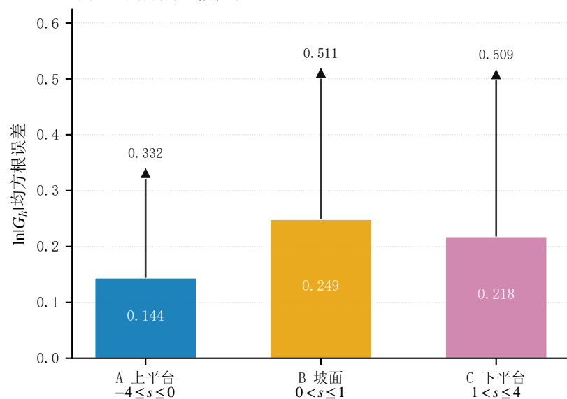
(d) 空间分层：幅值误差
