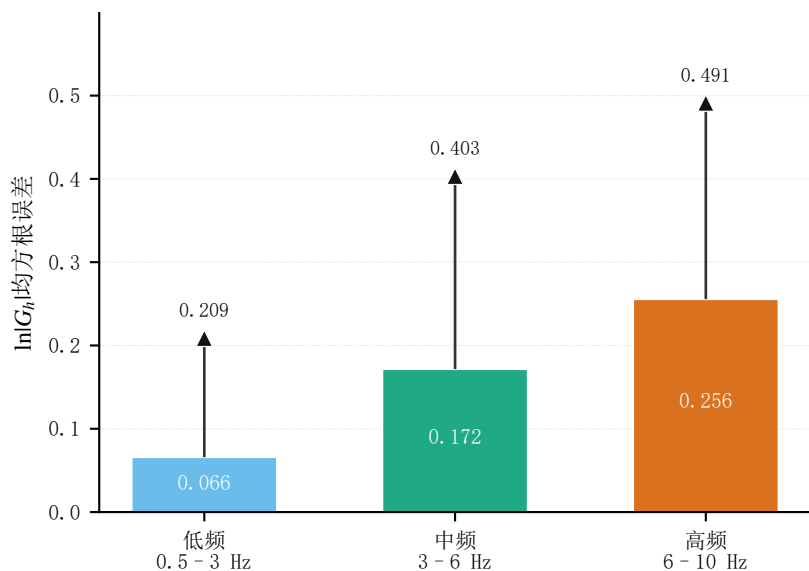
(a) 频带分层：幅值误差
