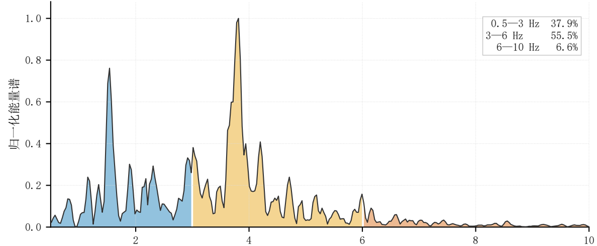
(b) 0.5—10 Hz能量分布
