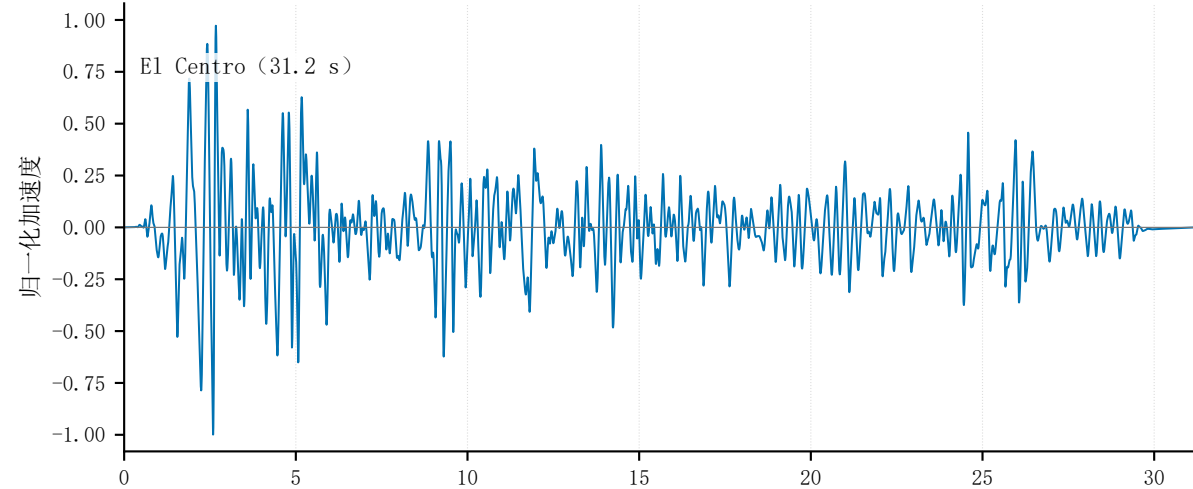
(a) 左侧上平台一维自由场时程
