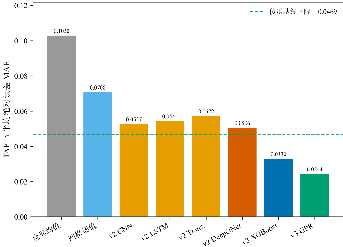
(a) TAF_h 全方法误差对照
