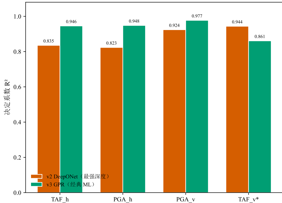
(b) 四通道 R^2 对照
