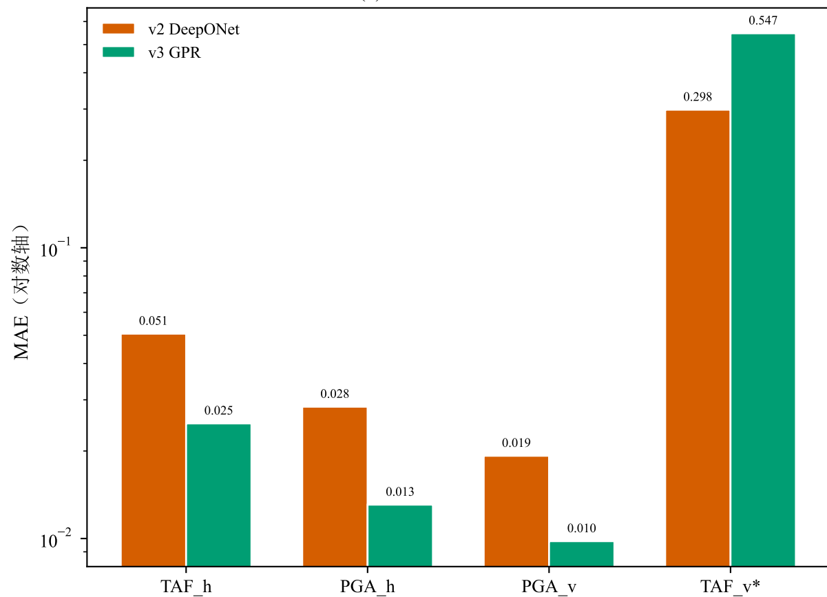
(c) 四通道 MAE 对照
