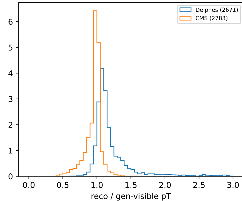
gen pT 30-50 GeV
