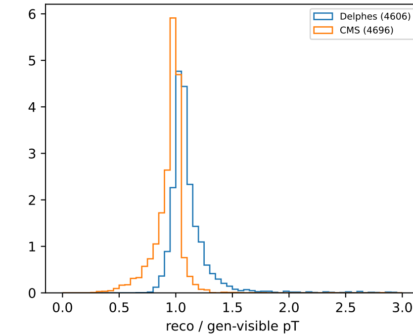
gen pT 50-100 GeV
