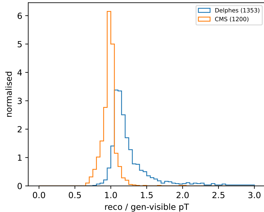
gen pT 20-30 GeV
