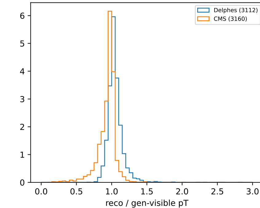
gen pT 100-300 GeV
