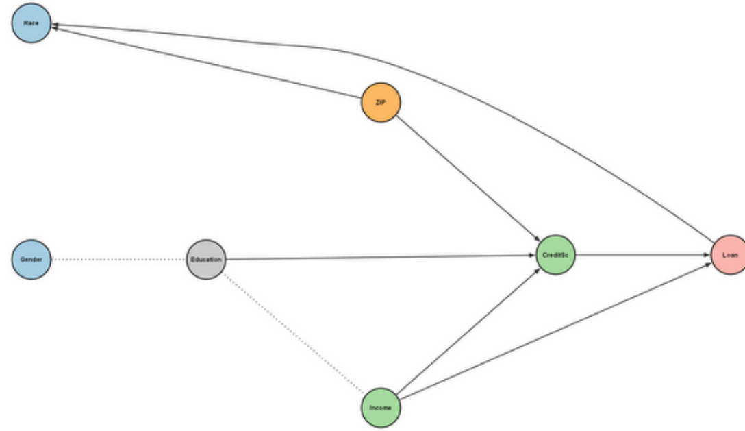
PC
