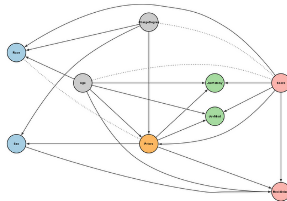
GES
