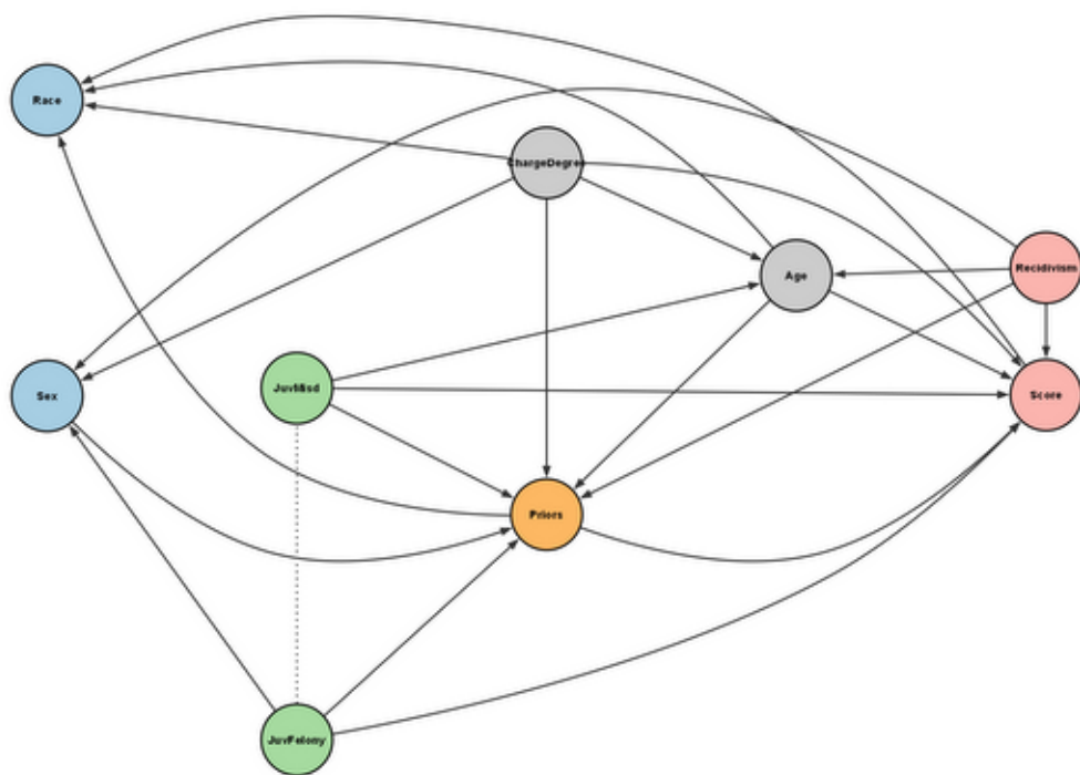
PC
