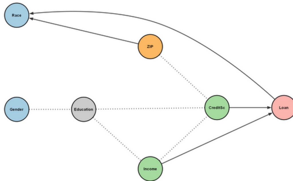
FCI
