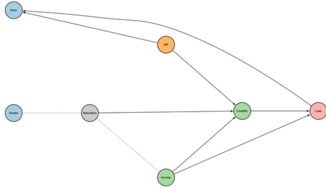
PC
