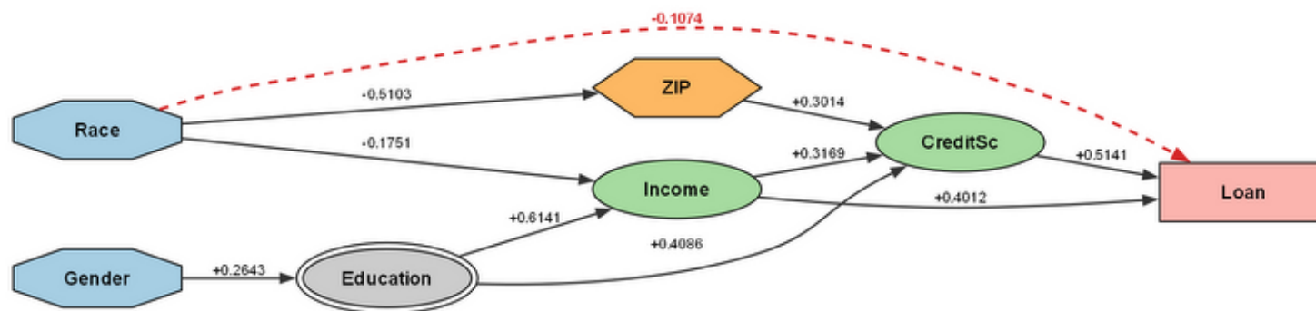
DirectLiNGAM est. \beta = -0.1074
