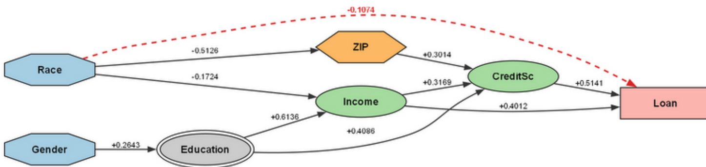
ICA-LiNGAM est. \beta = -0.1074
