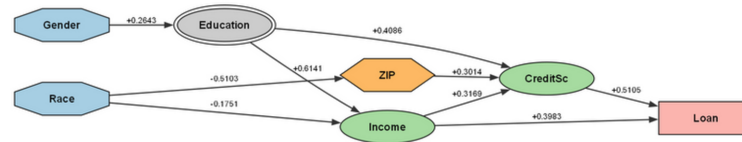
DirectLiNGAM est. \beta = +0.0000
