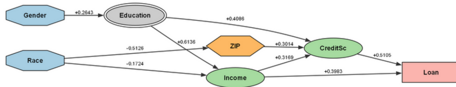
ICA-LiNGAM est. \beta = +0.0000
