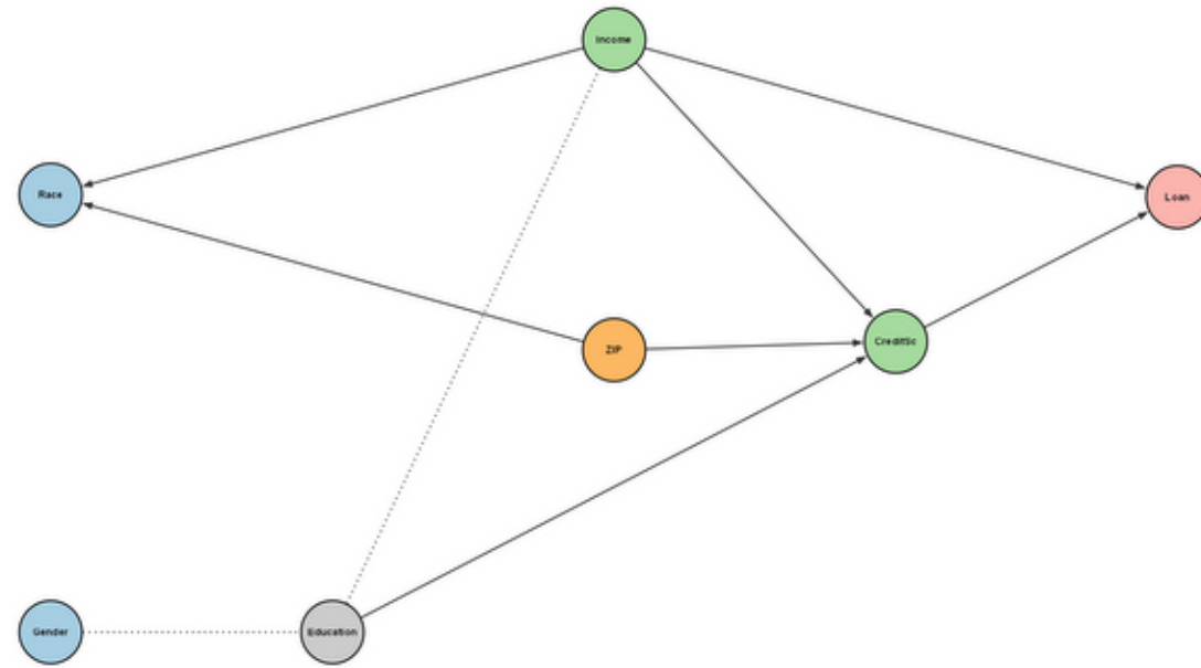
PC
