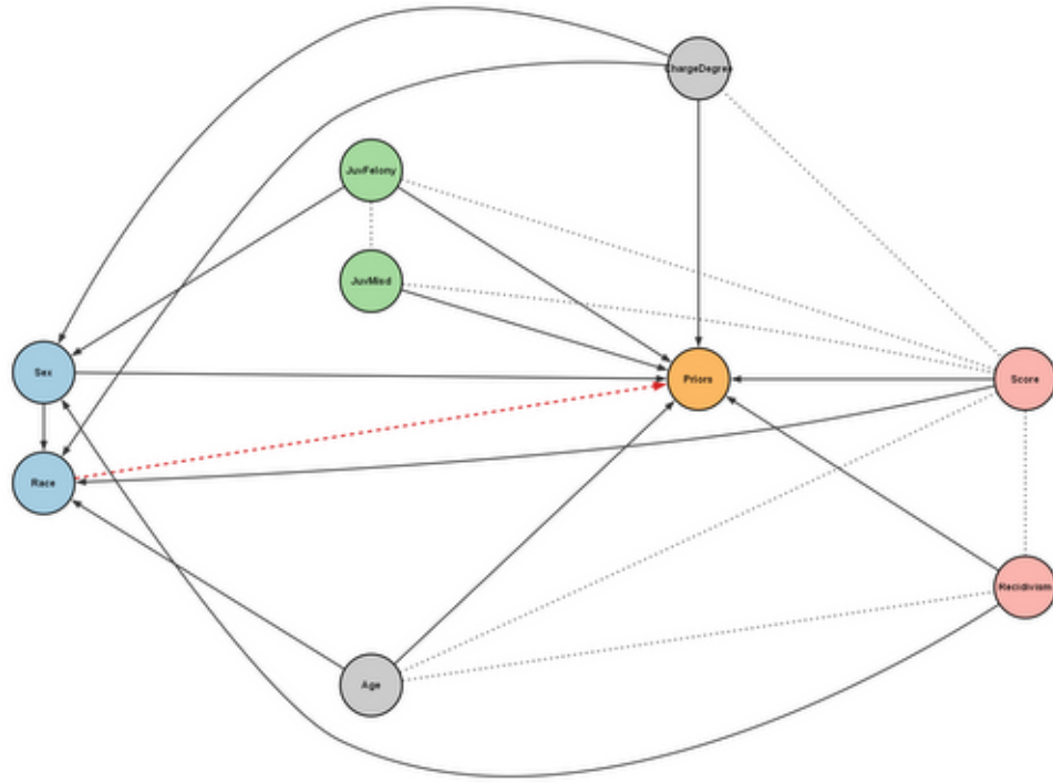
PC
