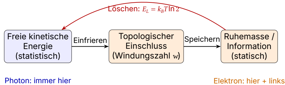
Abbildung ag.1: Zweiteilung der Energie in FFGFT. Freie kinetische Energie (blau) kann durch topologischen Einschluss in statische Masse/Information (orange) überführt werden. Das Löschen (roter Pfeil) setzt die eingefrorene Energie als Wärme frei – Landauers Prinzip. Das Photon verbleibt dauerhaft im kinetischen Sektor.
