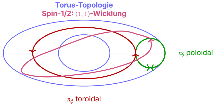
Abbildung al.1: Spin-1/2 als topologische Wicklung auf dem Torus (Draufsicht). Der grüne Doppelpfeil zeigt den poloidalen kleinen Kreis ( n_\theta , Querschnitt des Torus-Schlauchs). Die roten Pfeile zeigen die toroidale Richtung ( n_\phi , um das zentrale Loch). Der violette Pfad zeigt eine (1,1)-Wicklung: einmal um den kleinen Kreis UND einmal um den großen Kreis. Eine 720^\circ -Rotation entspricht zweimaligem Durchlaufen dieser Wicklung.
