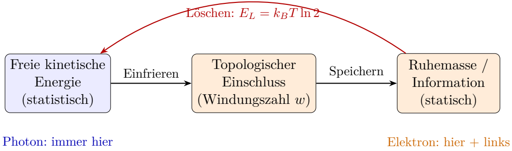
Abbildung 1: Zerteilung der Energie in FFGFT. Freie kinetische Energie (blau) kann durch topologischen Einschluss in statische Masse/Information (orange) überführt werden. Das Löschen (roter Pfeil) setzt die eingefrorene Energie als Wärme frei – Landauers Prinzip. Das Photon verbleibt dauerhaft im kinetischen Sektor.
