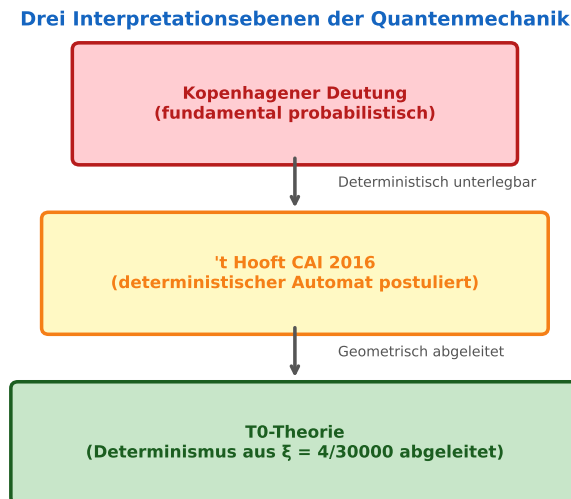
Abbildung 1: Drei Interpretationsebenen der Quantenmechanik: Kopenhagener Deutung (probabilistisch), CAI von 't Hooft (Automat postuliert), T0-Theorie (Determinismus aus \xi abgeleitet). Jede Ebene subsumiert die vorherige.
