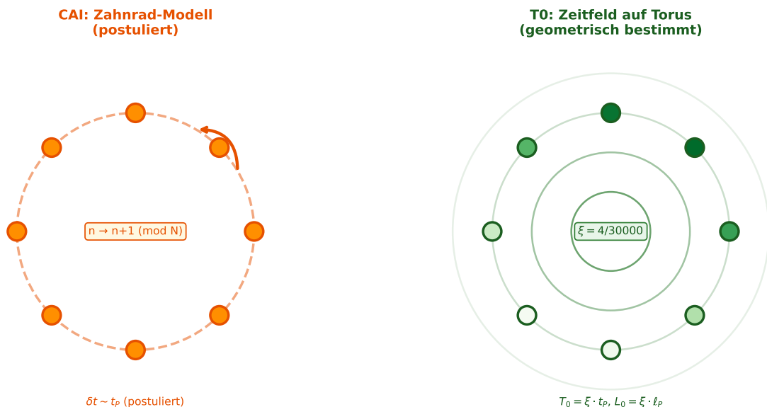
Abbildung 2: Links: CAI-Zahnrad mit N = 8 diskreten Zuständen (postulierte Struktur). Rechts: T0-Zeitfeld T(x, t) auf geometrischem Torus mit L_0 = \xi \cdot \ell_P (abgeleitete Struktur).
