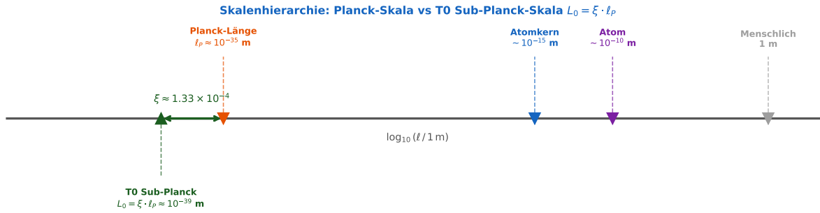
Abbildung 5: Skalenhierarchie von der menschlichen Skala bis zur T0 Sub-Planck-Skala. Die T0-Gitterkonstante L_0 = \xi \cdot \ell_P liegt um den Faktor \xi \approx 1,33 \times 10^{-4} unterhalb der Planck-Länge.
