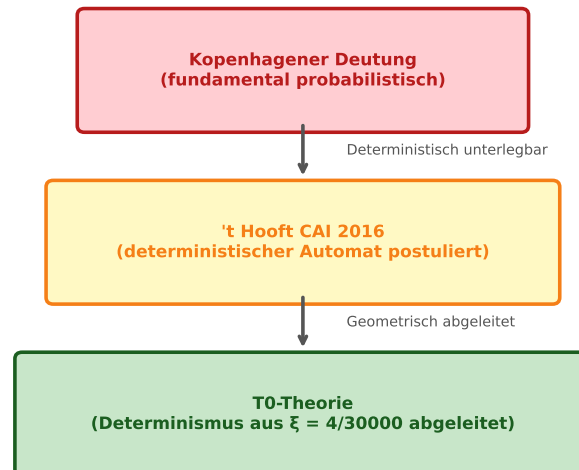
Abbildung 1: Drei Interpretationsebenen der Quantenmechanik: Kopenhagener Deutung (probabilistisch), CAI von 't Hooft (Automat postuliert), T0-Theorie (Determinismus aus \xi abgeleitet). Jede Ebene subsumiert die vorherige.
