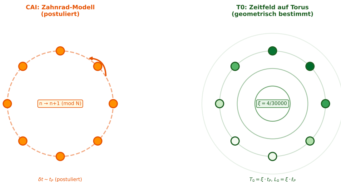
Abbildung 2: Links: CAI-Zahnrad mit N = 8 diskreten Zuständen (postulierte Struktur). Rechts: T0-Zeitfeld T(x, t) auf geometrischem Torus mit L_0 = \xi \cdot \ell_p (abgeleitete Struktur).
