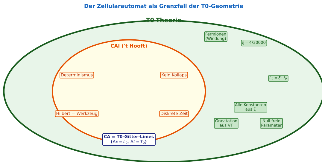
Abbildung 3: Inklusionsdiagramm: Die CAI (orange) ist als Grenzfall in der T0-Theorie (grün) enthalten. Die äußeren grünen Elemente sind T0-Beiträge jenseits der CAI.
