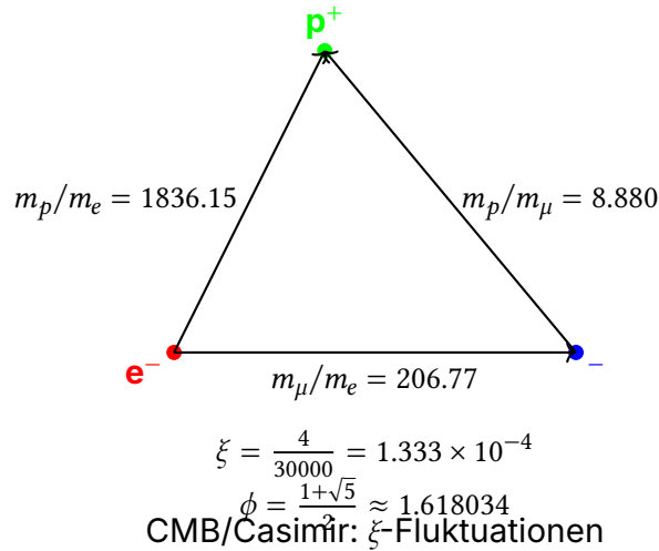
Abbildung 2.1: Fundamentales Massendreieck des e-p- \mu -Systems (erweitert um kosmologische \xi -Effekte)
