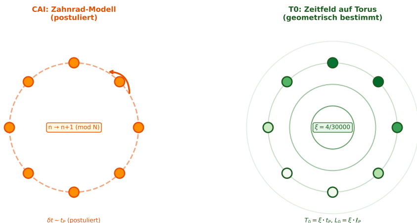
Abbildung S.2: Links: CAI-Zahnrad mit N = 8 diskreten Zuständen (postulierte Struktur). Rechts: T0-Zeitfeld T(x, t) auf geometrischem Torus mit L_0 = \xi \cdot l_p (abgeleitete Struktur).
