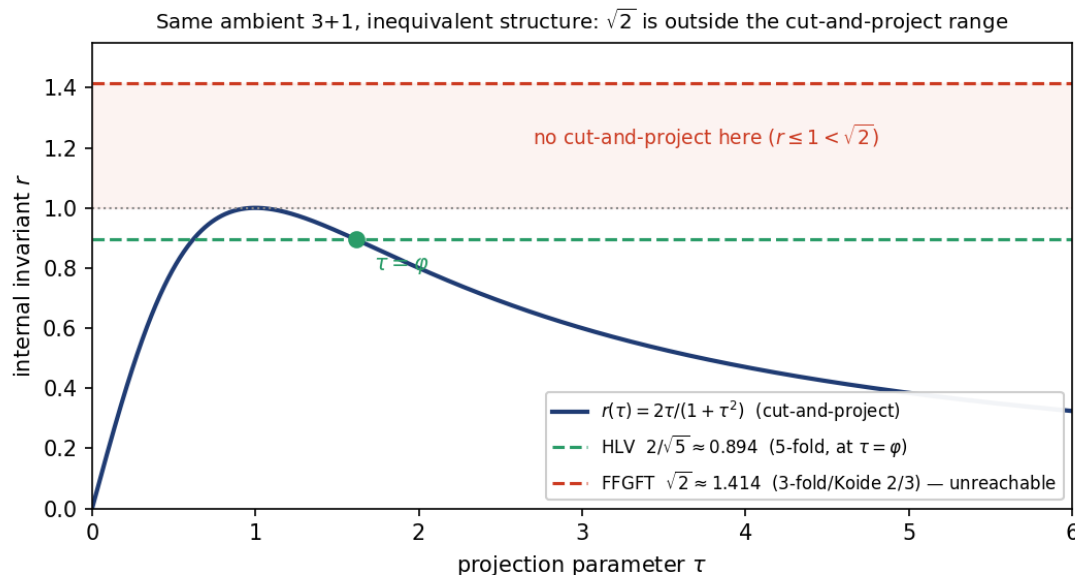
Abbildung T.1: Der cut-and-project-Invariant r(\tau) \leq 1 erreicht HLVs 2/\sqrt{5} bei \tau = \varphi , aber nie FFGFTs \sqrt{2} . Dass \sqrt{2} über dem Maximum dieser Familie liegt, heißt nur, dass diese eine Projektion die beiden Invarianten nicht ineinander überführt – nicht, dass die Strukturen unverträglich sind (siehe nächster Abschnitt).
