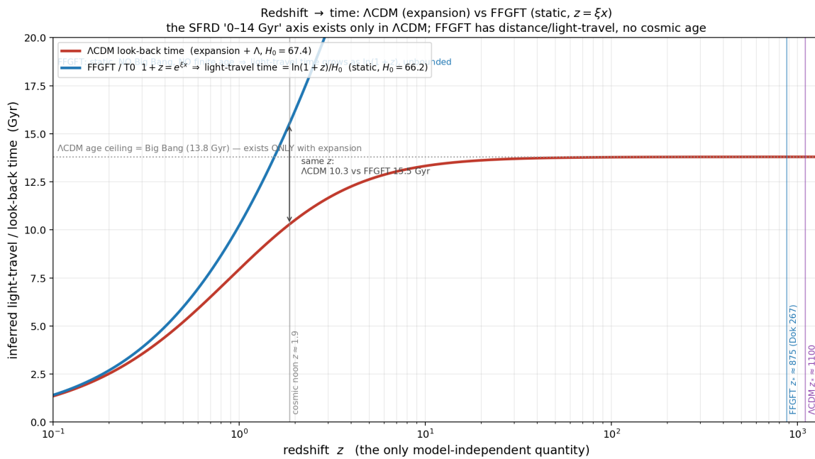
Abbildung O.1: Rotverschiebung \rightarrow Zeit ist modellabhängig. \Lambda CDM-Lookback (rot, Expansion + \Lambda ) saturiert bei der Urknall-Decke 13,8 Gyr; FFGFT (blau, statisch, 1 + z = e^{\xi x} ) liefert eine unbeschränkte Lichtlaufzeit \ln(1 + z)/H_0 ohne Urknall. Bei „cosmic noon“ ( z \approx 1,9 ): \Lambda CDM 10,3 vs. FFGFT 15,5 Gyr. Rekombination: \Lambda CDM z_* \approx 1100 , FFGFT z_* \approx 875 (Dok. 267).
