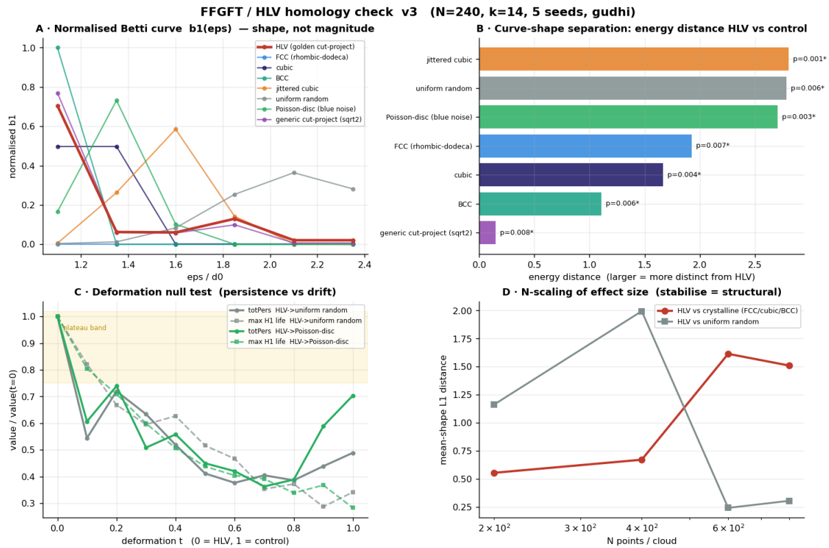
Abbildung L.1: Vier-Felder-Übersicht des Begleitskripts (v3). A: normierte Betti-Kurven b_1(\epsilon) – Form, nicht Betrag. B: Energie-Distanz der Kurvenform HLV gegen Kontrollen. C: Deformations-Null-Test (Gesamtpersistenz und, mit gudhi, längste H_1 -Lebensdauer). D: N-Skalierung der Effektstärke (stabil = strukturell). Endliche Diagnostik; keine Aussage über physikalische Raumzeit-Mikrostruktur.
