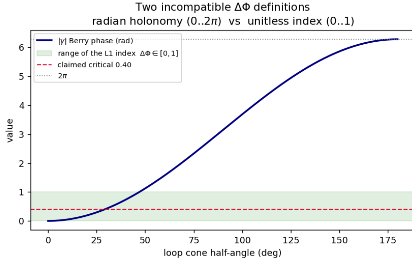
Abbildung S.2: Die zwei \Delta\Phi -Definitionen sind unvereinbare Objekte: eine Holonomie im Bogenmaß (0 ... 2\pi ) gegenüber einem einheitenlosen Index (0 ... 1).
