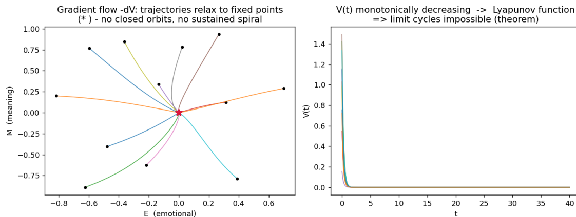
Abbildung S.3: Gradientenfluss mit den DLHR-Potenzialen des Papiers: Trajektorien relaxieren in Fixpunkte (keine geschlossenen Orbits, keine anhaltende Spirale), und V(t) fällt monoton, sodass Grenzzyklen unmöglich sind.
