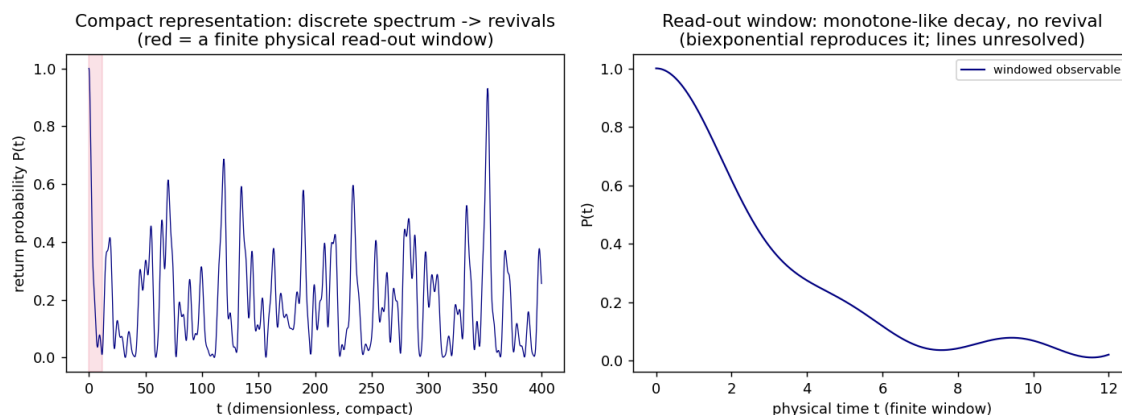
Abbildung S.1: Auslesung als nicht-invertierbare Projektion. Links: in der kompakten Darstellung erzeugt das diskrete Spektrum Wiederkehren (Back-flow \gg 0 ); das rote Band markiert ein endliches physikalisches Auslesefenster. Rechts: im Fenster zerfällt das Observable ohne Wiederkehr, und die diskreten Linien sind unaufgelöst.
