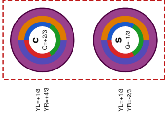
SU(2)_L -Dublett = Sd-Sektor [B] Dok.349
