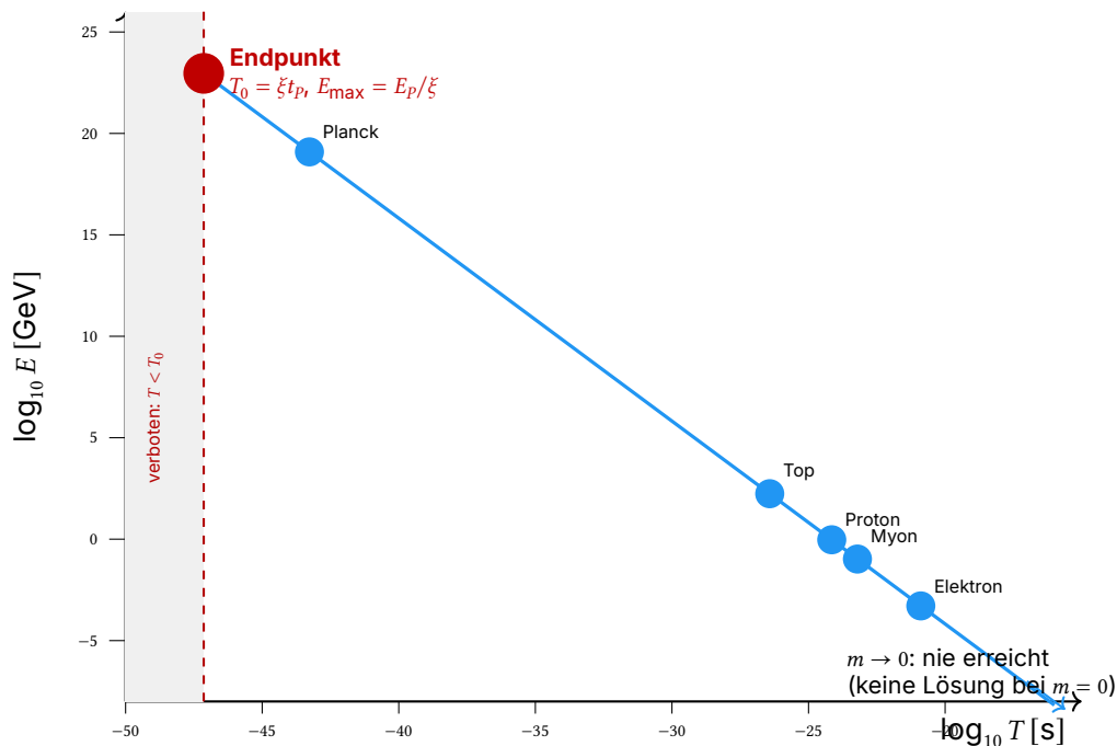
Abbildung ao.1: Die Relation T \cdot E = 1 (in SI: T \cdot E = \hbar ) in doppelt-logarithmischen Koordinaten: eine Gerade der Steigung -1 . Alle elementaren Anregungen liegen exakt auf ihr — keine ist ausgezeichnet, und die Gerade besitzt keine Mitte . Ausgezeichnet ist genau ein Punkt: der Endpunkt (T_0, E_{\max}) = (\xi t_P, E_P/\xi) , an dem die Kurve aufhört — die aus \xi folgende Wand. Am anderen Ende läuft sie als Asymptote weiter und kommt nie an ( T \cdot m = 1 hat bei m = 0 keine Lösung). Die beiden Ränder sind also verschiedenartig: links ein erreichter Endpunkt, rechts eine unerreichbare Grenze. Aufgetragen sind Skalen (Energie je Anregung), nicht Gesamtmassen; makroskopische Körper gehören nicht auf diese Achse.
