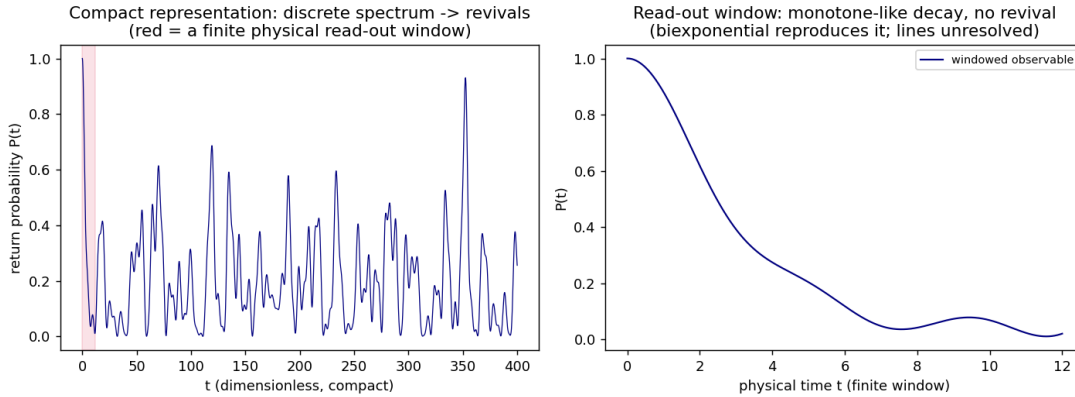
Abbildung S.1: Auslesung als nicht-invertierbare Projektion. Links: in der kompakten Darstellung erzeugt das diskrete Spektrum Wiederkehren ( \text{Back-flow} \gg 0 ); das rote Band markiert ein endliches physikalisches Auslesefenster. Rechts: im Fenster zerfällt das Observable ohne Wiederkehr, und die diskreten Linien sind unaufgelöst.
