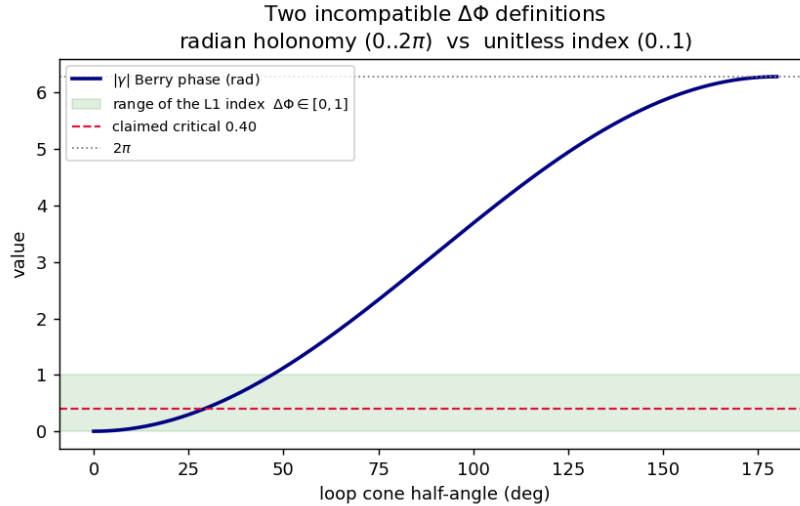
Abbildung S.2: Die zwei \Delta\Phi -Definitionen sind unvereinbare Objekte: eine Holonomie im Bogenmaß ( 0 \dots 2\pi ) gegenüber einem einheitenlosen Index ( 0 \dots 1 ).
