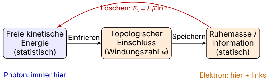
Abbildung af.1: Zerteilung der Energie in FFGFT. Freie kinetische Energie (blau) kann durch topologischen Einschluss in statische Masse/Information (orange) überführt werden. Das Löschen (roter Pfeil) setzt die eingefrorene Energie als Wärme frei – Landauers Prinzip. Das Photon verbleibt dauerhaft im kinetischen Sektor.
