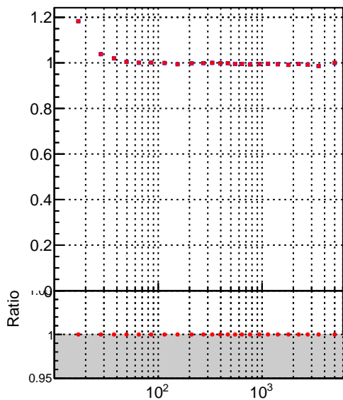
Jet pT response, eta=[0, 0.5]
