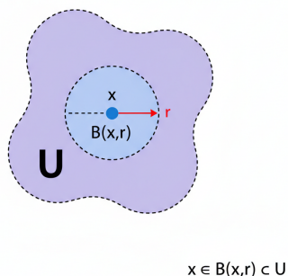
FIGURE 1.1 – Un ensemble U est un ouvert de la topologie forte si et seulement si chacun de ses points x peut être recouvert par une boule ouverte incluse dans U .
