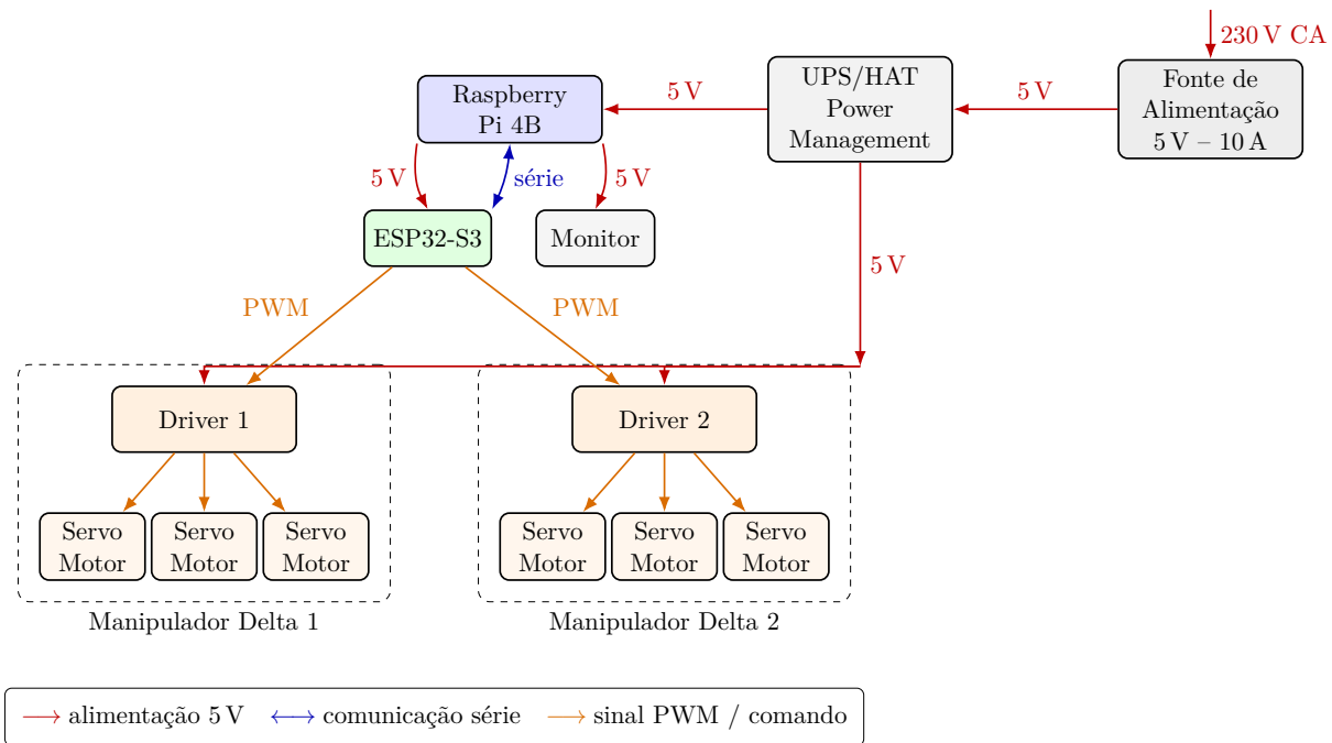
Figura 3.3: Esquema consolidado de alimentação, comunicação e comando dos dois manipuladores delta.
