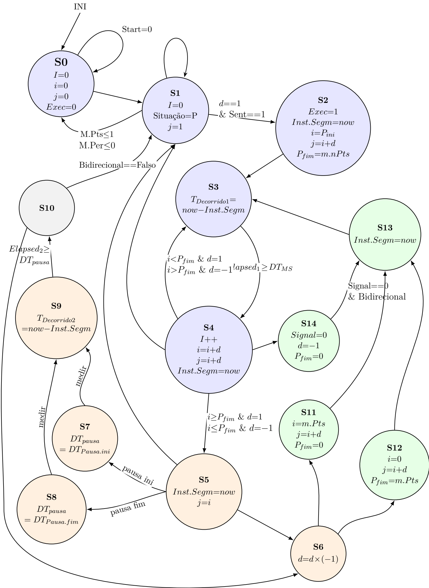
Figure 1: Esquema da FSM.Motion.Update.
