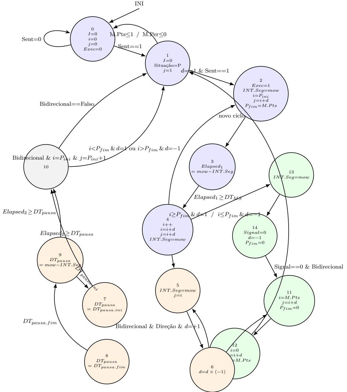
Figura 4.2: Esquema da FSM_Motion_Update.
