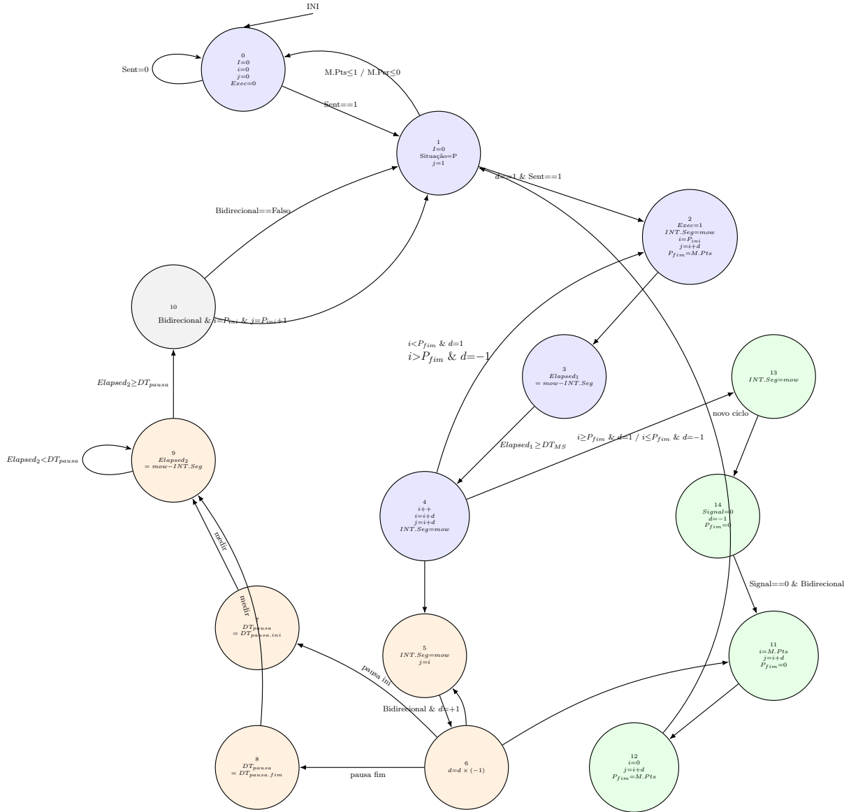
Figura 4.2: Esquema da FSM_Motion_Update.
