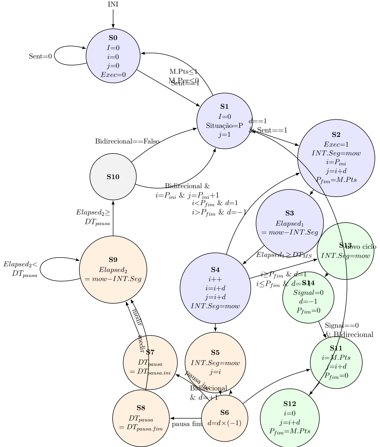
Figura 4.2: Esquema da FSM_Motion_Update.
