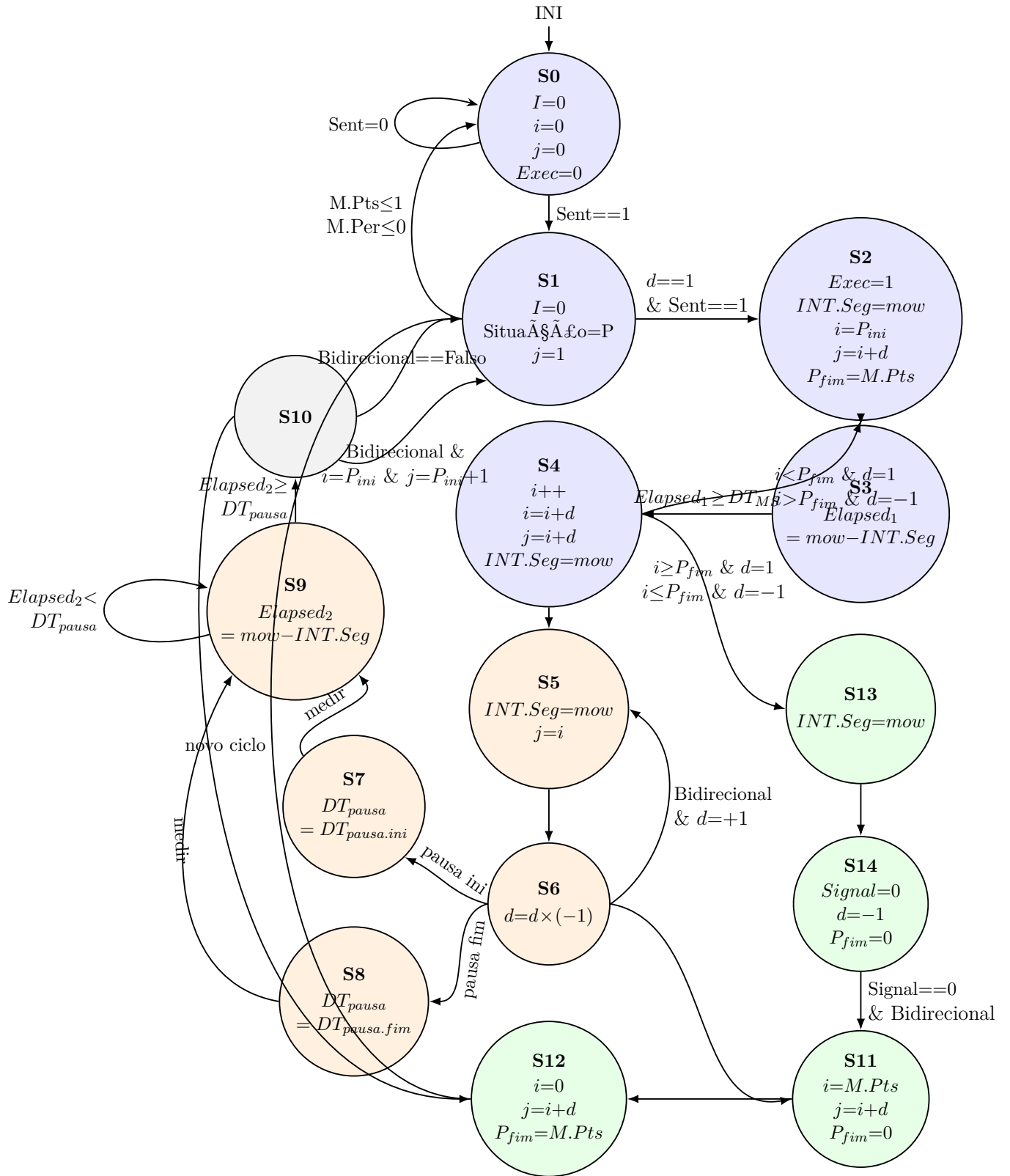
Figura 4.2: Esquema da FSM_Motion_Update.
