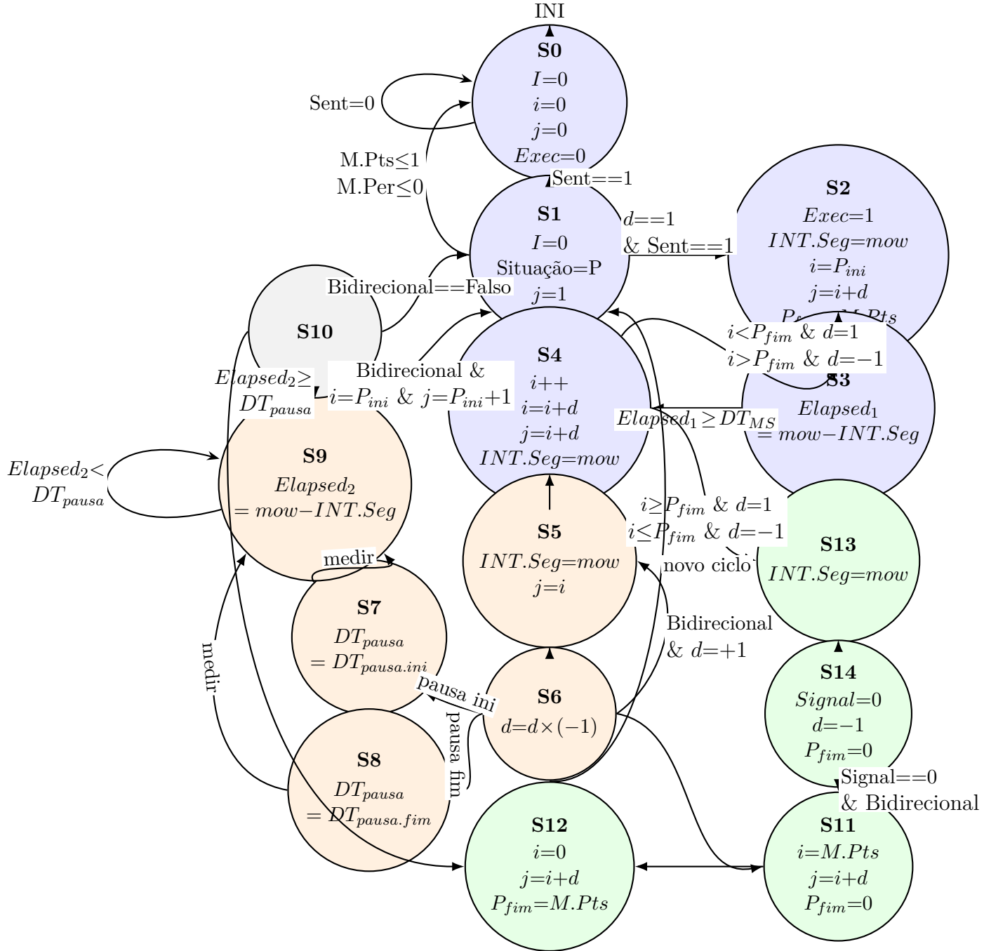
Figura 4.2: Esquema da FSM_Motion_Update.
